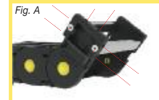
Fig. A NUOVO ATTACCO BASCULANTE 1- Diverse combinazioni di fissaggio. 2- Trafilato in alluminio con pettini fissacavo montato sia sul punto fisso che sul punto mobile. 3- Spazio creato per alloggiare dado.
