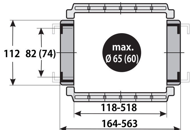
Размерные параметры в мм
