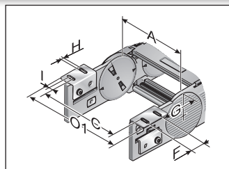
КА 66 (внеш. сторона вид сверху / снизу)
