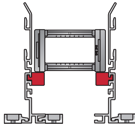
Сечение В-В: Энергоцепь скользит на профиле скольжения.
