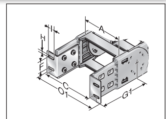
KA 62 (передняя сторона снаружи)
