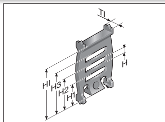
Разделительная перемычка открытая
