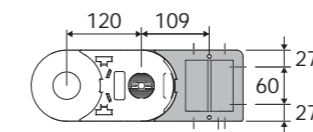
Fig. A La catena può essere fissata frontalmente sia interno che esterno raggio. (Fig A)
